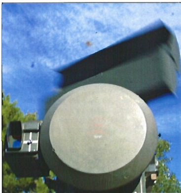
Radar de adquisición y seguimiento de la dirección de tiro
