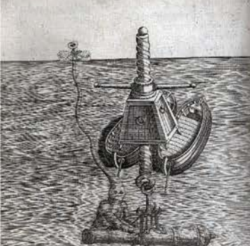
FIGURA DEL INSTRUMENTO EMPLEADO PARA SACAR PIEZAS DE ARTILLERIA DEL AGUA.
