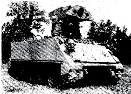
TOW sobre M 901, transporte acorazado de personal, perfeccionado.
