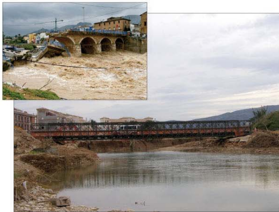
El montaje del puente Bailey duró cuatro días; arriba, el puente destruido
