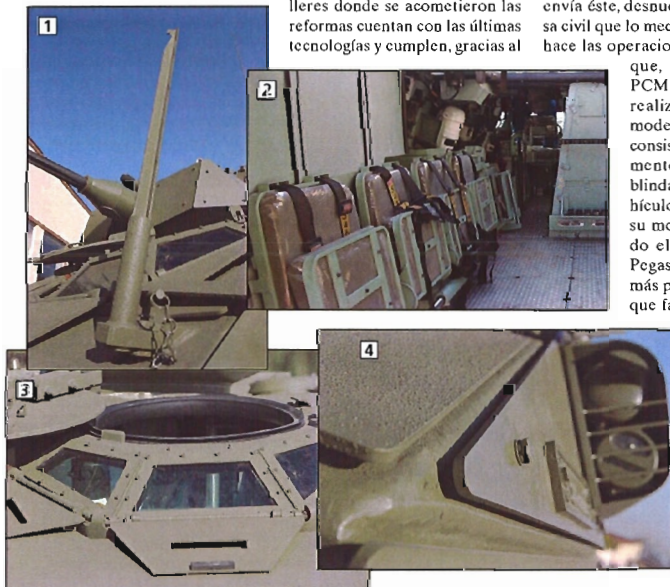
1) "Cortacables" del VEC. 2) Interior de un BMR; se aprecian los nuevos asientos y el Spectronix —la bombona blanca al fondo—. 3) Nueva cúpula del VEC. 4) Blindaje adicional
