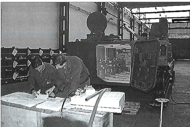
Técnicos de la factoría SBB, en Sevilla, verifican sobre los planos los cambios realizados en el último prototipo del Pizarro.
