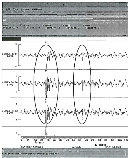
Registro sísmológico de dos pruebas indias, a principios de mayo.
