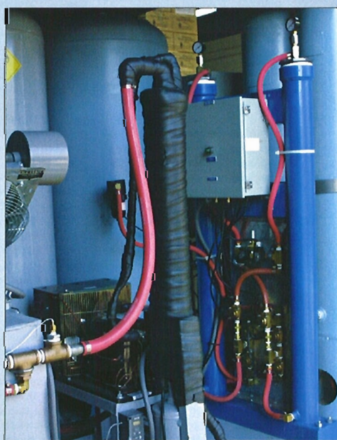
Secador-refrigerador (izquierda) y lechos de zeolita (derecha)
