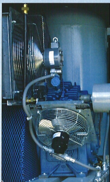
Compresor que recoge el aire
